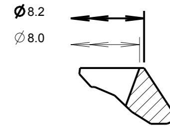
SECTION A-A SCALE 12:1
